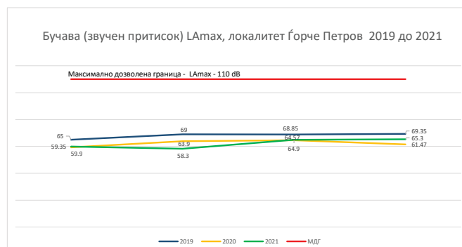
Графикон бр. 22 Мерења бучава (звучен притисок Ld и LAmax), локалитет Ѓорче Петров, за 2021 и за споредбениот период од 2019 до 2021 г.
